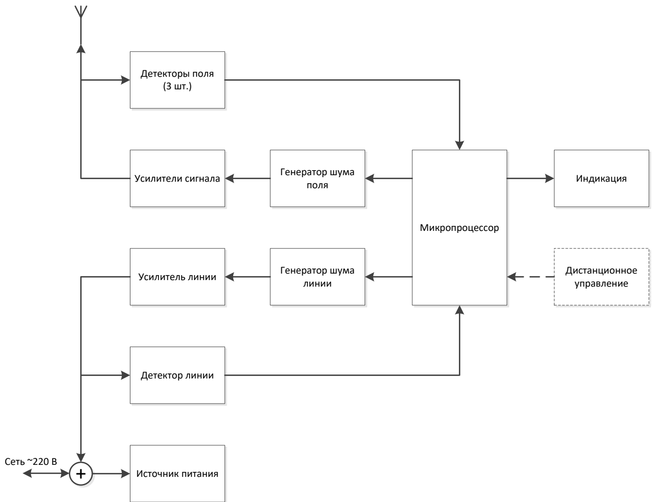
Рисунок 1 – Функциональная схема
